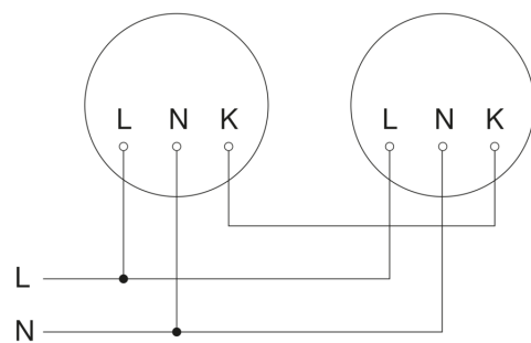
aansluitschema master/master
